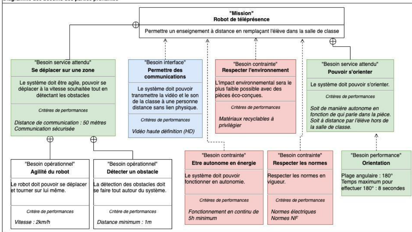
Diagramme des besoins des parties prenantes
